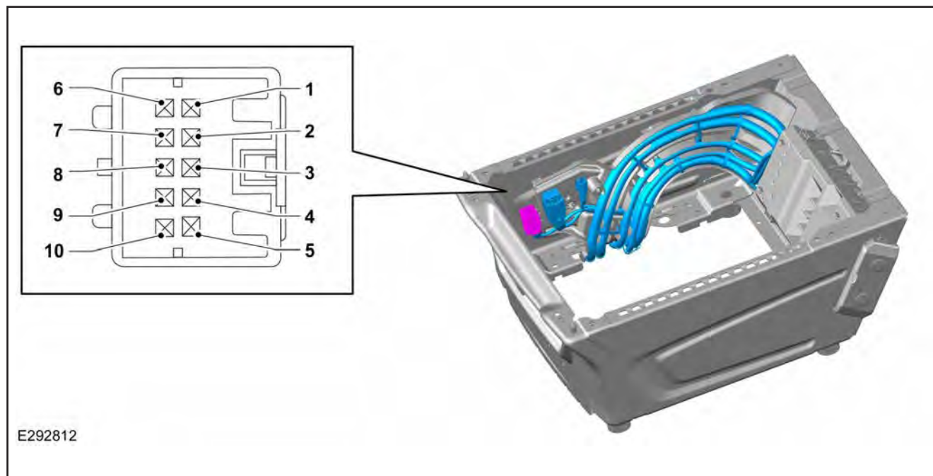
Sinais do conector de interface do veículo de 10 vias
